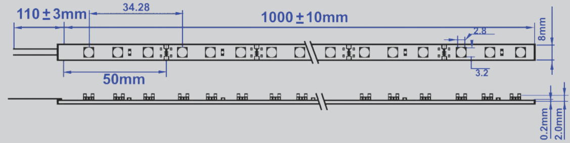
Şerit Led Detayı Led Strip Detail
