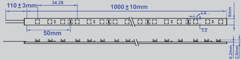
Şerit Led Detayı Led Strip Detail
