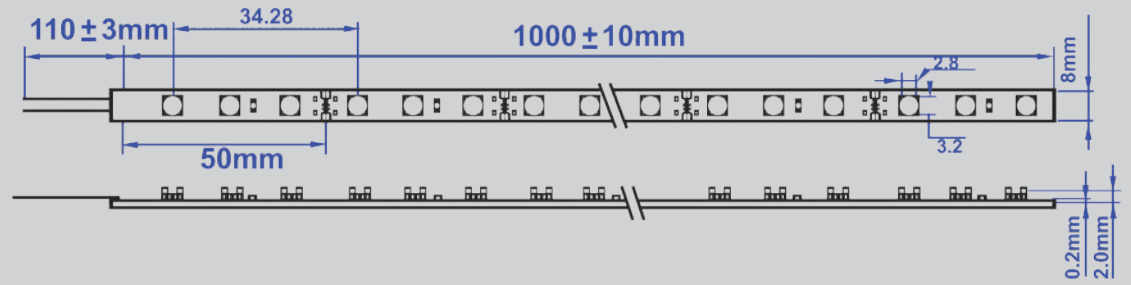
Şerit Led Detayı Led Strip Detail
